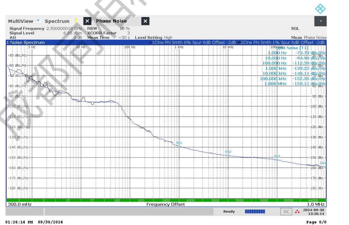
2500MHz 相位噪声测试图
